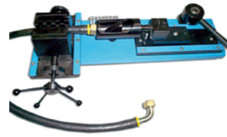
Introdutor rápido para racores Manual nipple inserter
